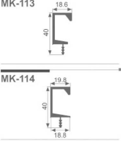
露边G型拉手 Dew and G type shake handshandle 颜色:黄铜拉丝、哑黑、星空灰、 星空黑、博洛尼红、哑铁灰、咖啡金 适用18-25mm板
