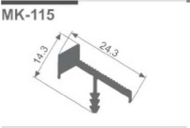
菱形斜边拉手 Diamond hypotenuse shake handshandle 颜色:黄铜拉丝、哑黑、星空灰、 星空黑、博洛尼红、哑铁灰、咖啡金 适用18mm板
