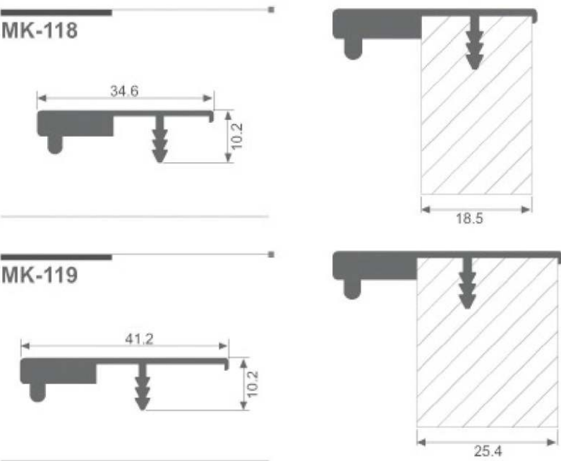
T型拉手 T shape handshandle 颜色:黄铜拉丝、哑黑、星空灰、 星空黑、博洛尼红、哑铁灰、咖啡金 适用18-25mm板
