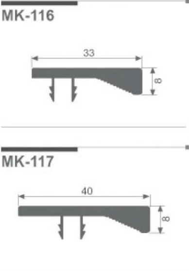
F型卡玻璃拉手 F type glass handle 颜色:黄铜拉丝、哑黑、星空灰、 星空黑、博洛尼红、哑铁灰、咖啡金 适用25mm板
