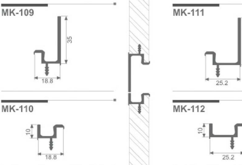
子母全盖拉手 Lash cover all shake handshandle 颜色:黄铜拉丝、哑黑、星空灰、 星空黑、博洛尼红、哑铁灰、咖啡金 适用18mm板/25mm板
