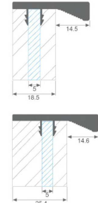
F型卡玻璃拉手 F type glass handle 颜色:黄铜拉丝、哑黑、星空灰、 星空黑、博洛尼红、哑铁灰、咖啡金 适用25mm板
